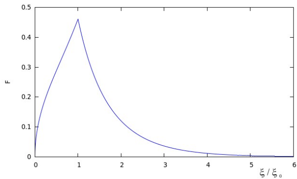
Fig 12 Solución en función de \xi/\xi_0
