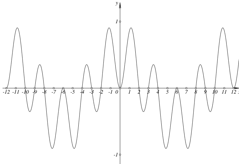
FIGURE 1.1 – Graphe de la fonction S_3
