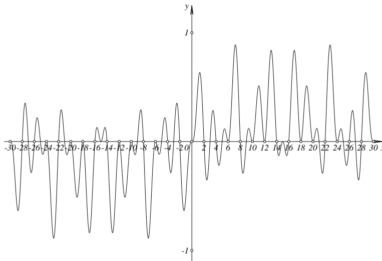
FIGURE 1.2 – Graphe de la fonction S_5
