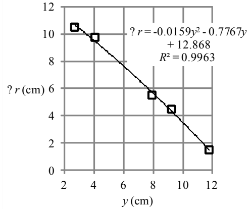
Gambar 8. Jarak antara titik puncak kurva parabola dengan posisi intruder \Delta r sebagai fungsi posisi vertikal intruder y .
