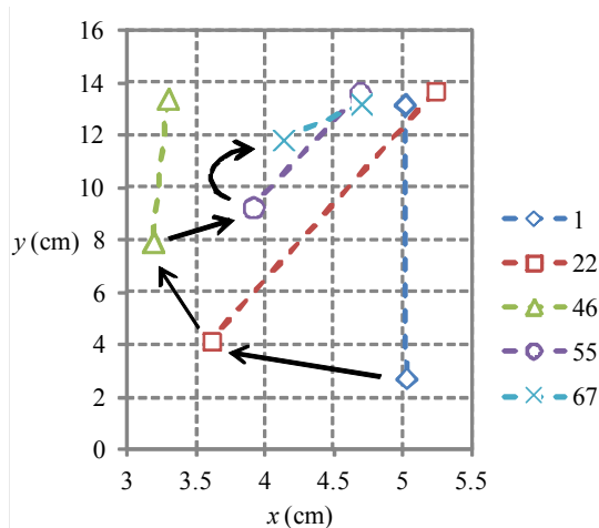
Gambar 7. Kaitan antara posisi intruder dengan posisi puncak dari kurva parabola untuk konfigurasi 1, 22, 46, 55, dan 67.
