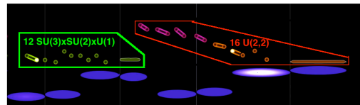
8 Fermion AntiParticles
