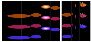
M4 M4 x CP2 Kaluza-Klein Quaternionic Spacetime
