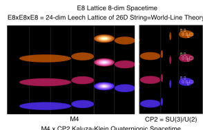
M4 M4 x CP2 Kaluza-Klein Quaternionic Spacetime
