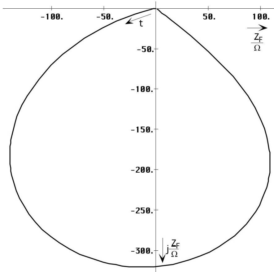
Bild 28 Ortskurve des Feldwellenwiderstands
