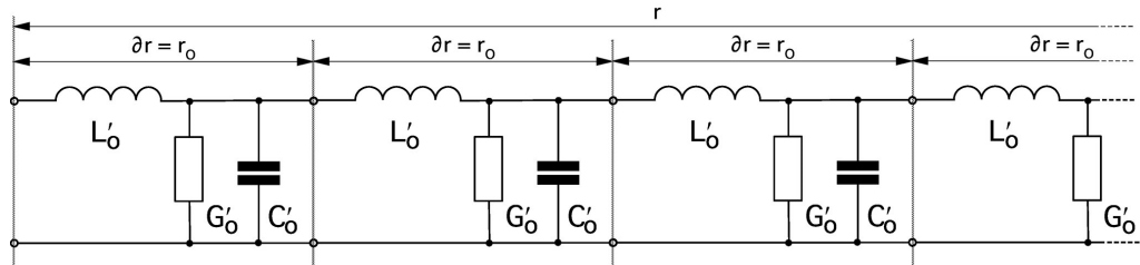
Bild 33 Leitungersatzschaltung mit Parallelleitwert
