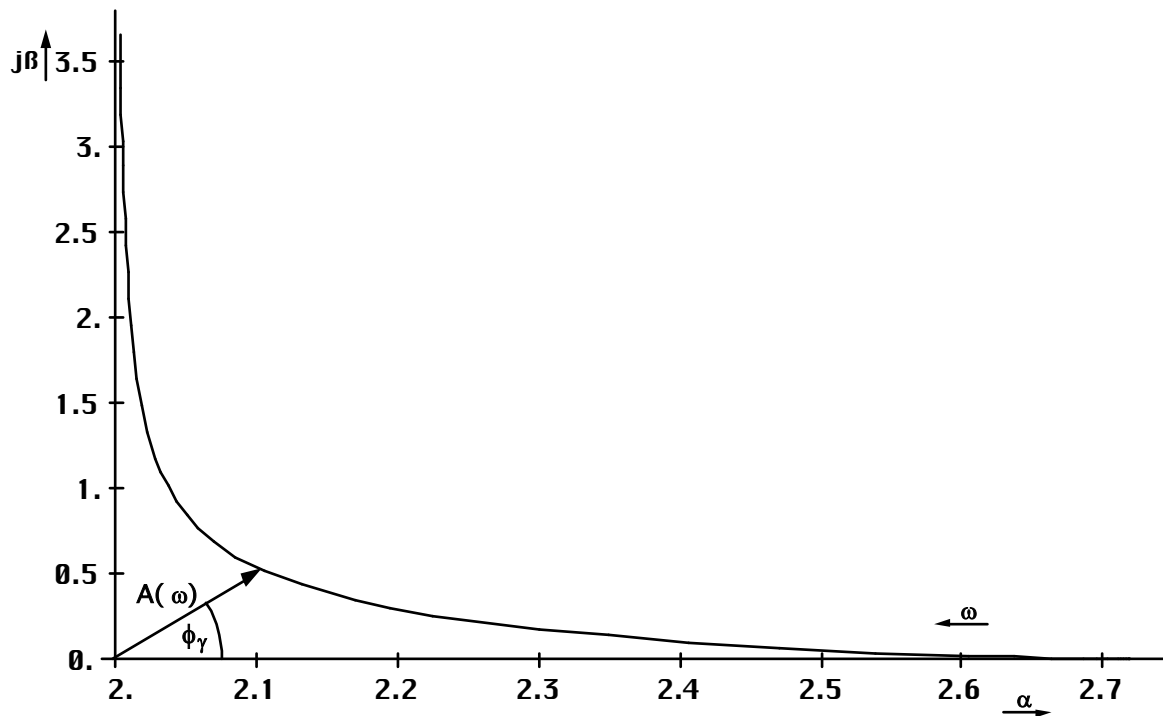
Bild 16 Frequenzgangsortskurve
