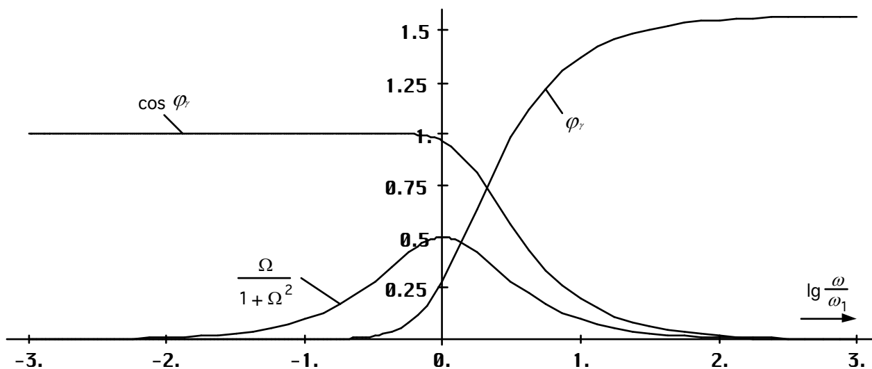
Bild 18 Verlauf von Phasenwinkel, \cos \phi und des Ausdrucks \frac{\Omega}{1 + \Omega^2}
