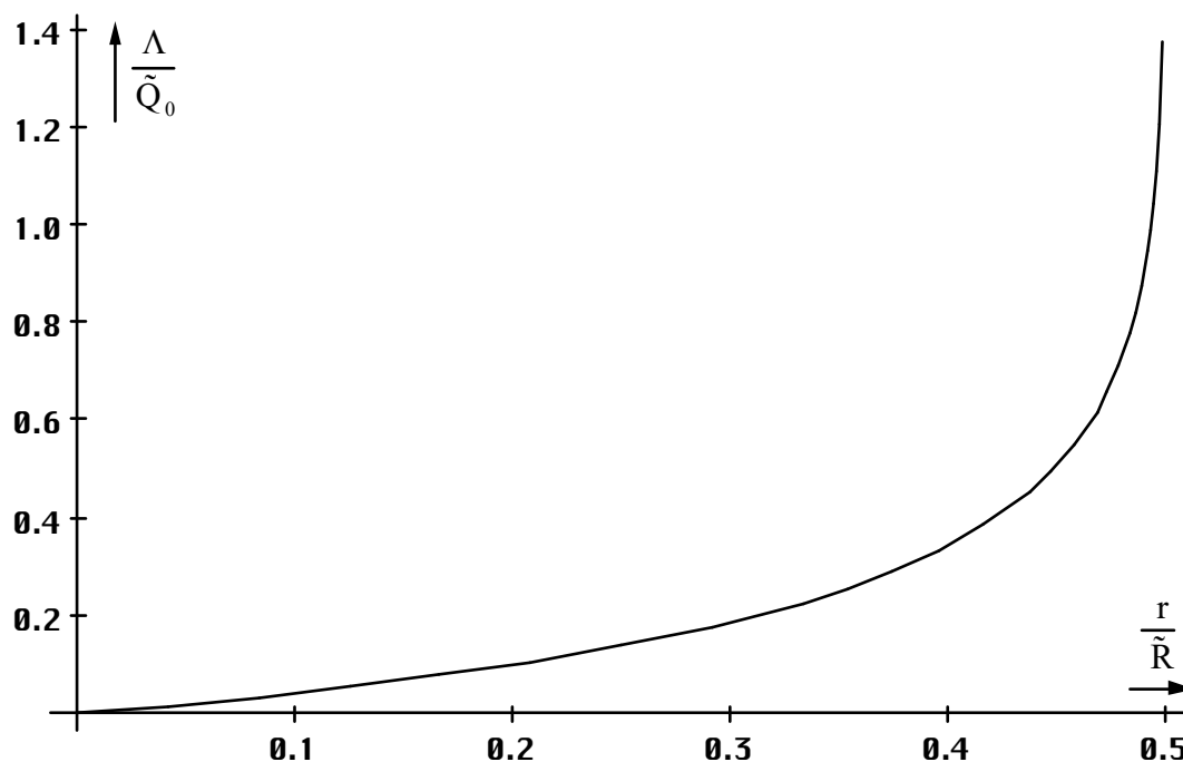
Bild 37 Wellenzahlvektor als Funktion des Abstands für t=0
