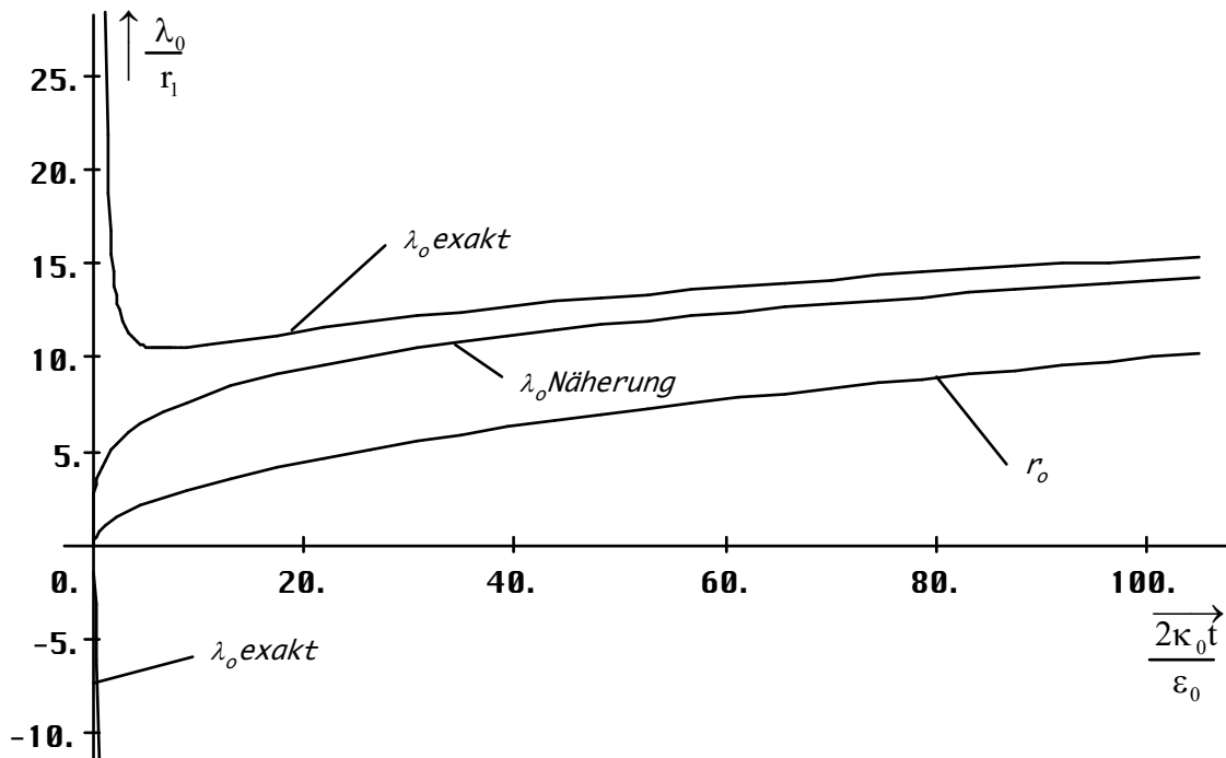
Bild 31 Verlauf von \lambda_0 \text{ exakt} und Näherung sowie r_0 linearer Maßstab
