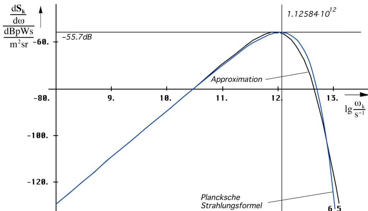
Bild 68 PLANCKSche Strahlungsformel und Approximation
