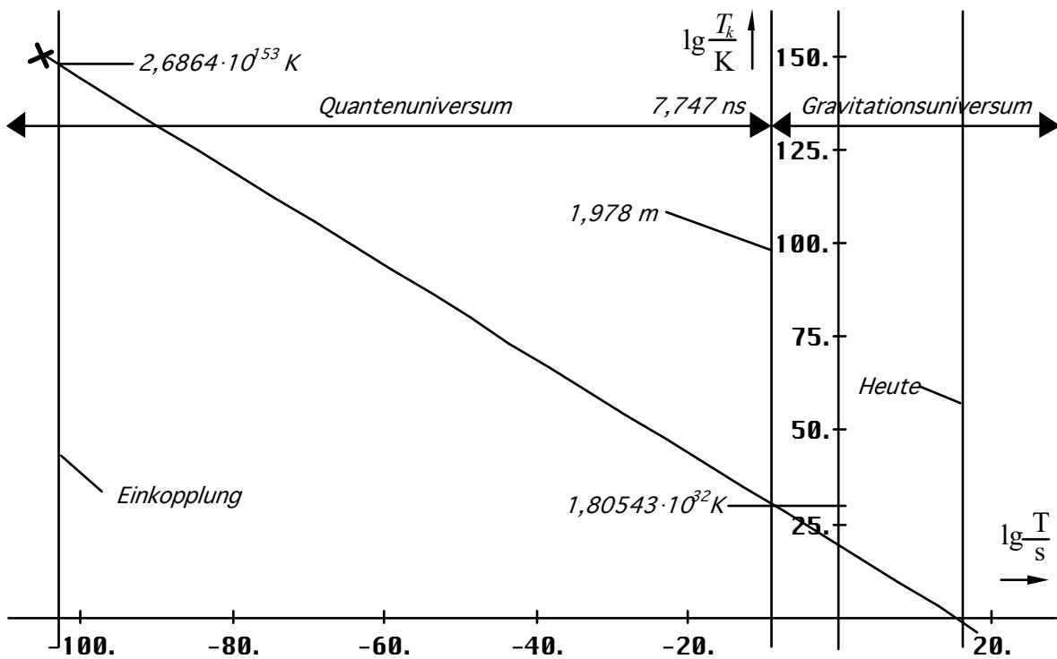
Bild 76 Zeitliche Abhängigkeit der Strahlungstemperatur der kosmischen Hintergrundstrahlung vom Zeitpunkt der Einkopplung an betrachtet
