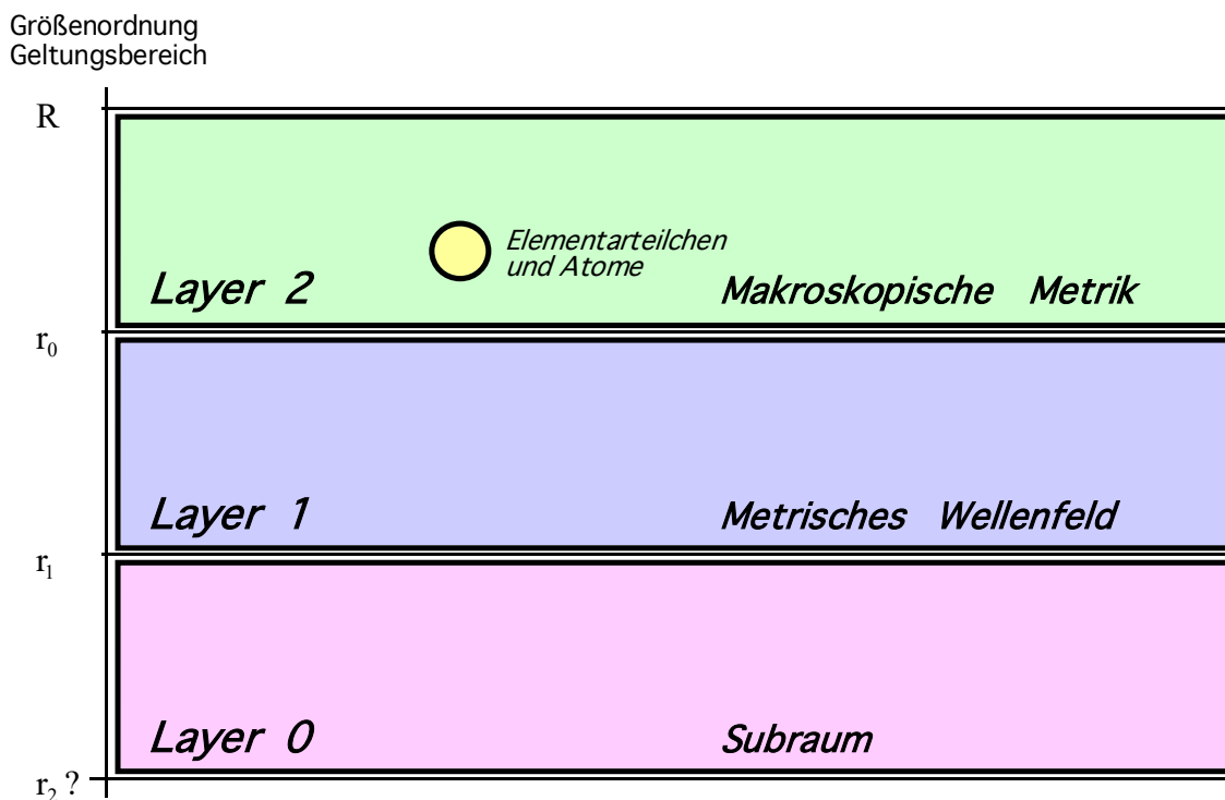
Bild 136 Das 3-Schichten-Modell der Metrik
