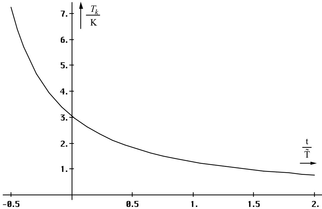
Bild 75 Zeitliche Abhängigkeit der Strahlungstemperatur der kosmischen Hintergrundstrahlung (linear)
