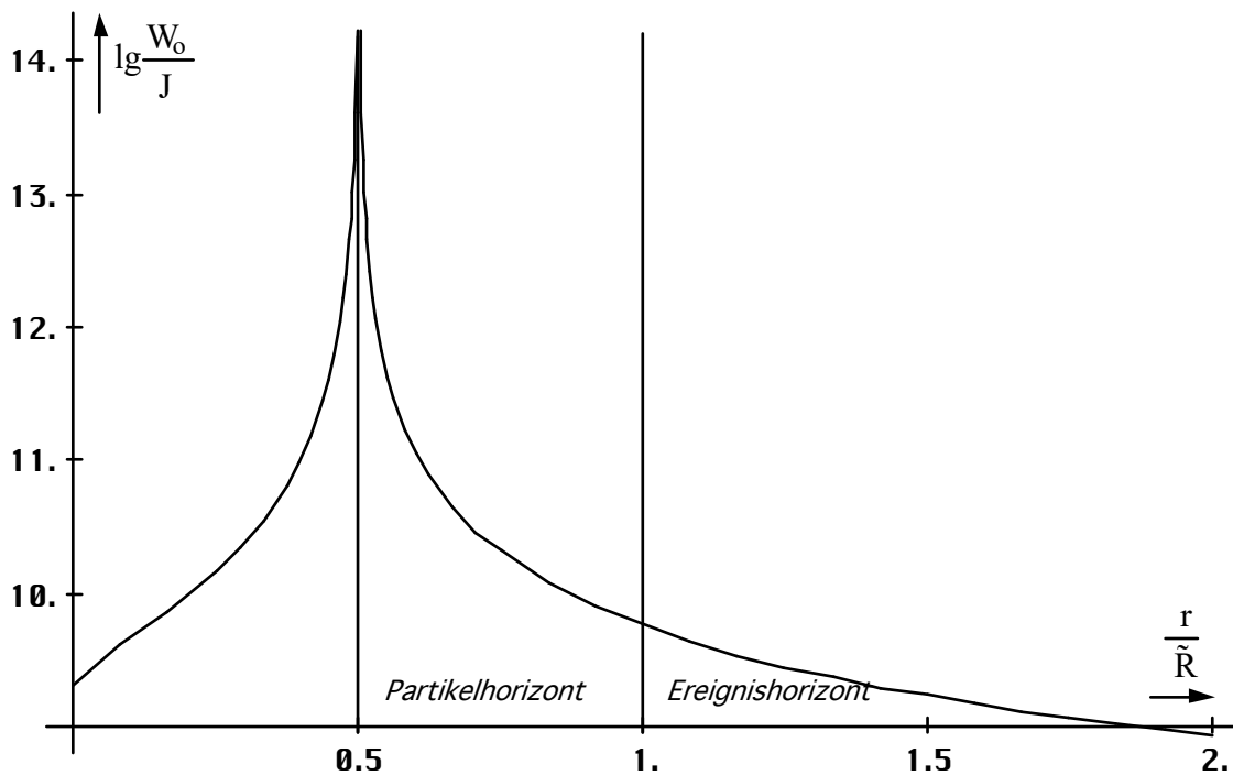
Bild 60 Energie des MINKOWSKISCHEN LINIELEMENTS räumliche Abhängigkeit am Partikelhorizont
