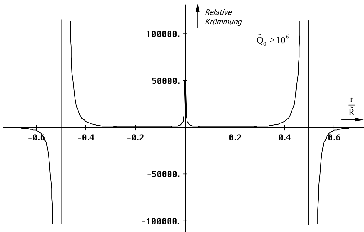
Bild 134 Relative skalare Krümmung für den Standardfall Q_0 > 10^6
