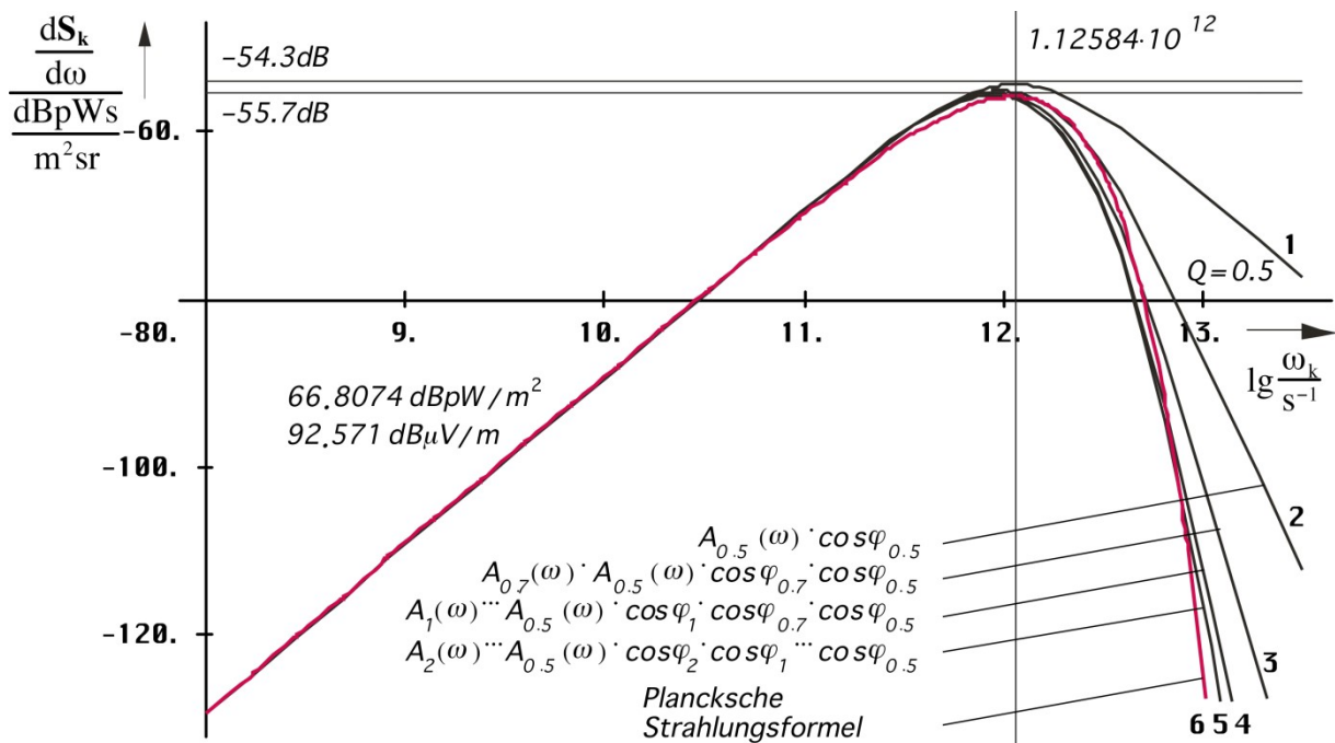
Bild 67 Intensität der kosmischen Hintergrundstrahlung mit Approximation
