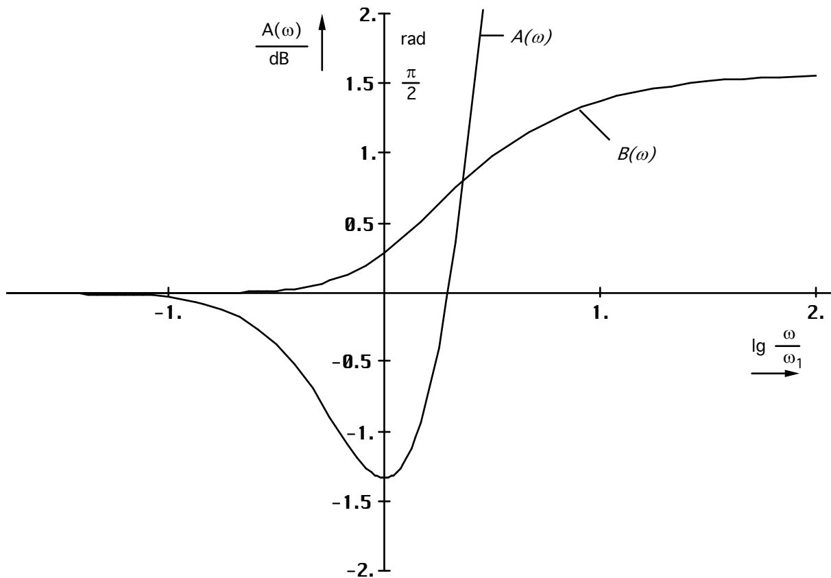
Bild 17 BODE-Diagramm: Frequenzgang A(\omega) und Phasengang B(\omega) des Systems
