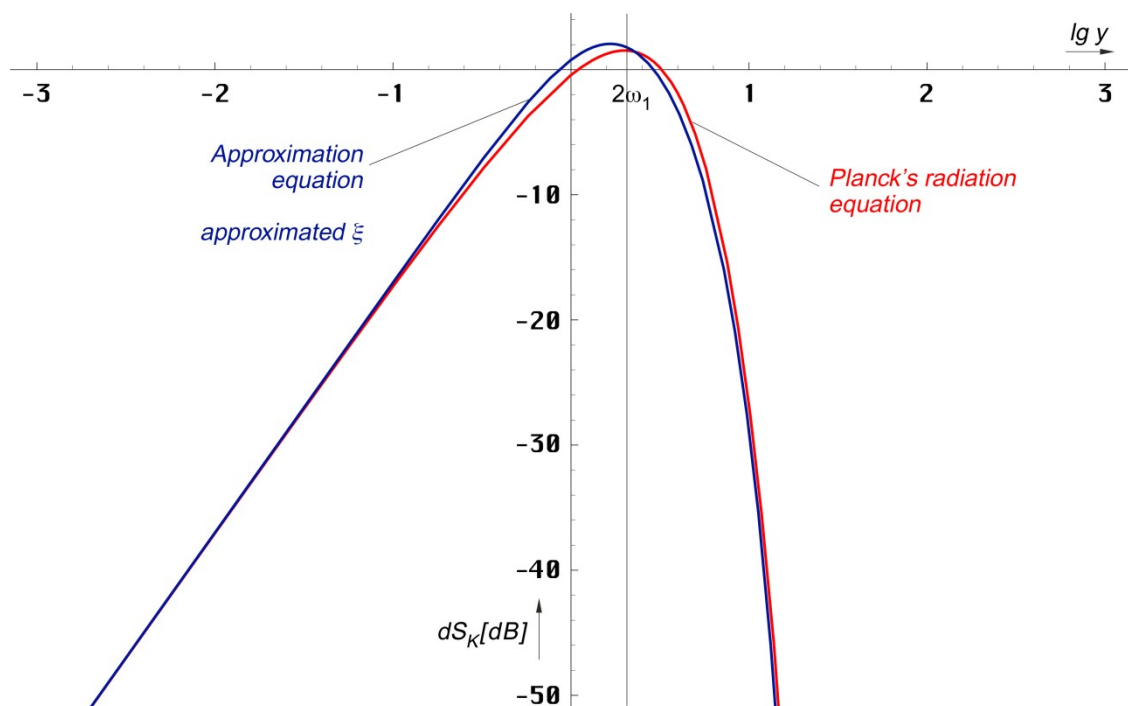
Bild 3 PLANCKS Strahlungsformel und Approximation mit Näherung für die Funktion \xi (relativer Pegel)
