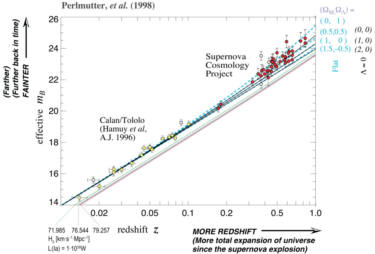
Bild 146 Berechnete scheinbare bolometrische Helligkeit für die drei Werte des HUBBLE-Parameters im Vergleich mit den Beobachtungen des Supernova-Kosmologie-Projekts (Standardkerze = Maximum)
