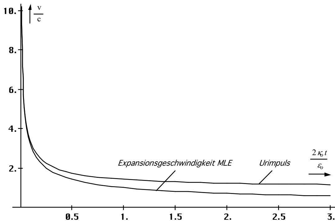
Bild 89 Ausdehnungsgeschwindigkeit von Uripuls und MINKOWSKISCHEM Linienelement Nr. 1
