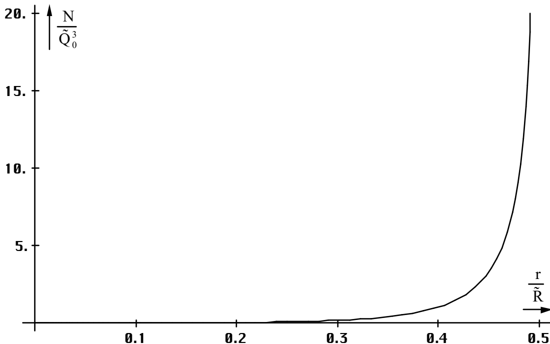
Bild 47 Anzahl MLE's in Abhängigkeit vom Radius
