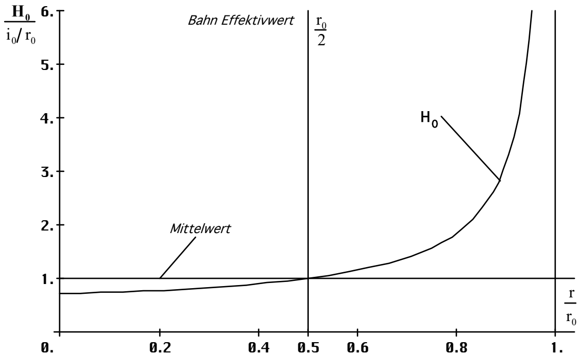
Bild 5 Verlauf der magnetischen Feldstärke in Abhängigkeit vom Radius r
