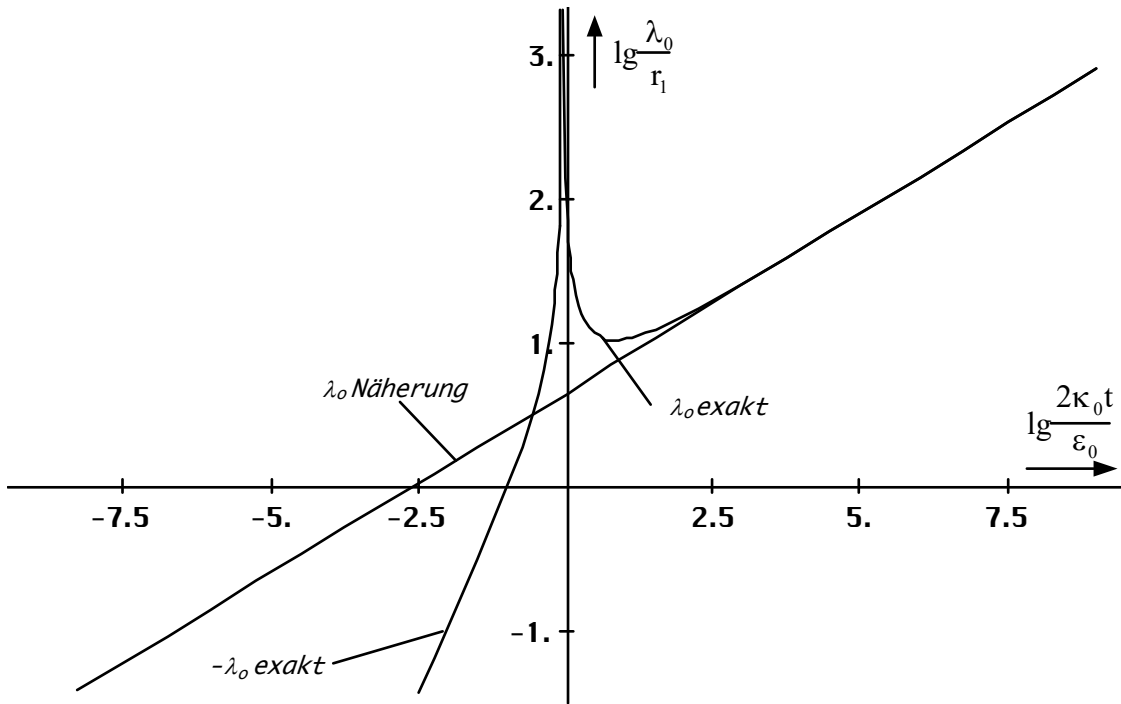
Bild 30 Verlauf von \lambda_0 \text{ exakt} logarithmischer Maßstab
