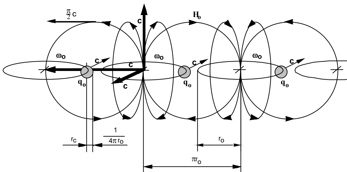
Bild 2 MINKOWSKISCHE Linienelemente Abmessungen und Kopplung untereinander
