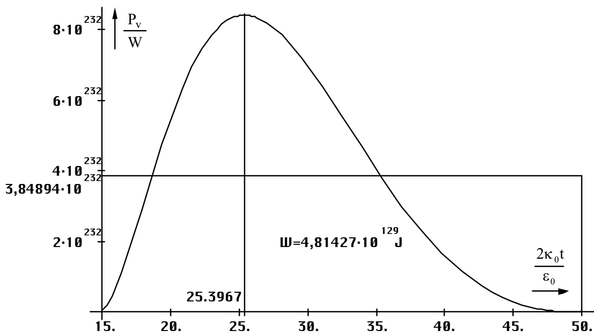
Bild 64 Verlustleistung des MINKOWSKISCHEN Linielements während des zweiten Maximums
