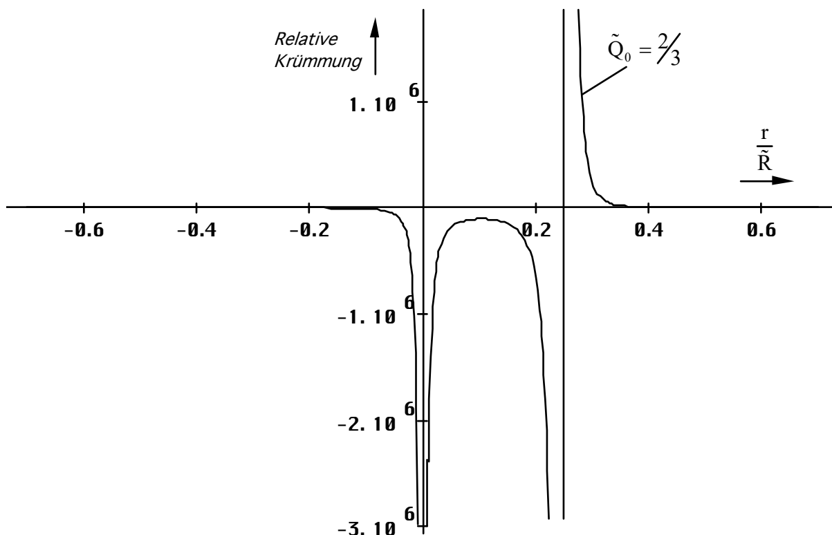
Bild 135 Relative skalare Krümmung für den Fall Q_0 = 2/3
