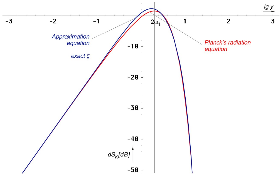
Bild 4 PLANCKS Strahlungsformel und Approximation unter Verwendung der exakten Funktion \xi (relativer Pegel)
