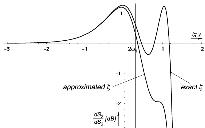
Bild 5 Relative Abweichung zwischen Approximation und Strahlungsformel in Abhängigkeit von der verwendeten Funktion \xi
