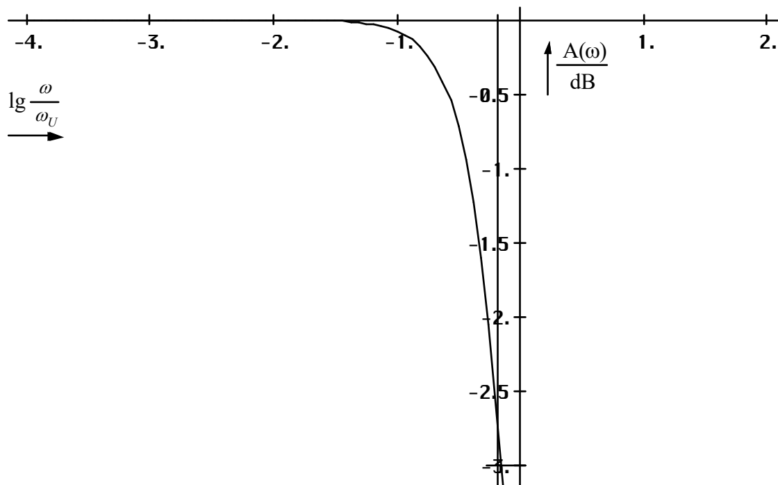
Bild 86 Normierte Spektralfunktion der elektrischen bzw. magnetischen Feldstärke des Urimpulses (logarithmischer Maßstab)
