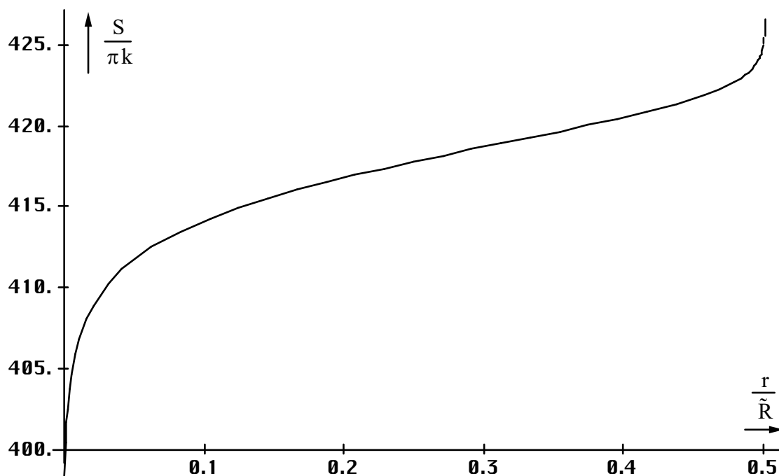
Bild 48 Entropie in Abhängigkeit vom Radius
