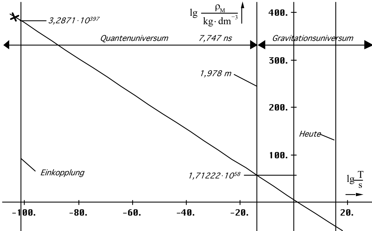
Bild 70 Zeitliche Abhängigkeit der mittleren Materiedichte vom Zeitpunkt der Einkopplung an betrachtet
