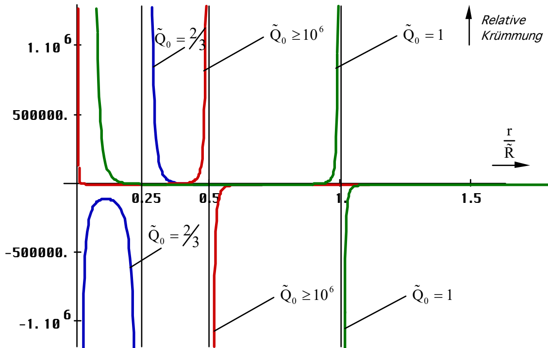
Bild 133 Relative skalare Krümmung für verschiedene Ausgangsgütwerte
