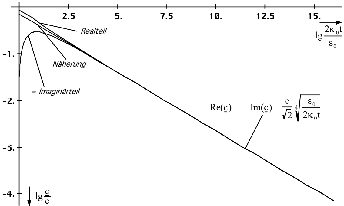
Bild 29 Ausbreitungsgeschwindigkeit in Abhängigkeit von der Zeit (logarithmisch)
