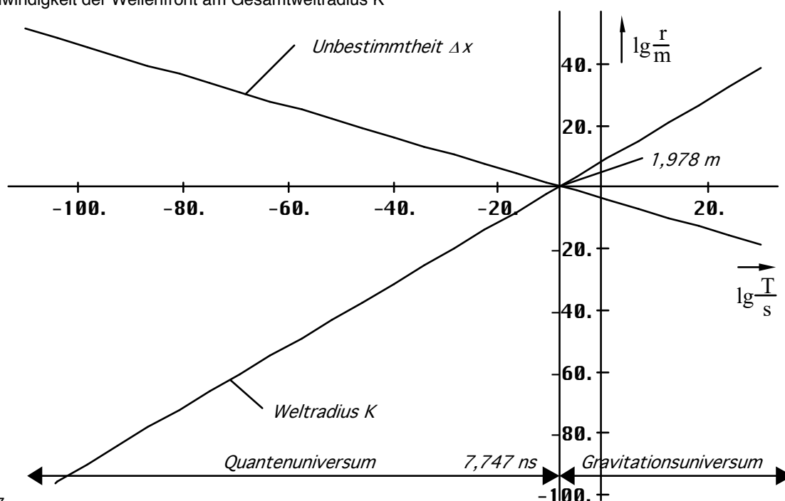
Bild 57 Quantenuniversum und Gravitationsuniversum
