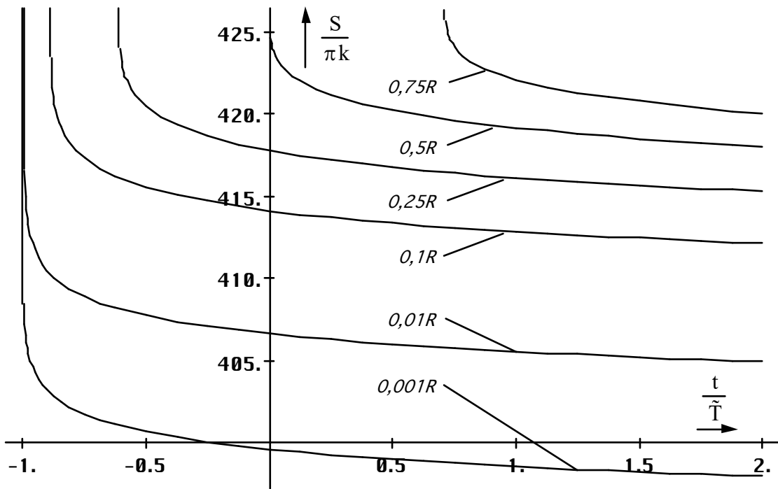
Bild 49 Zeitliche Abhängigkeit der Entropie für r=\text{const} (linearer Maßstab)
