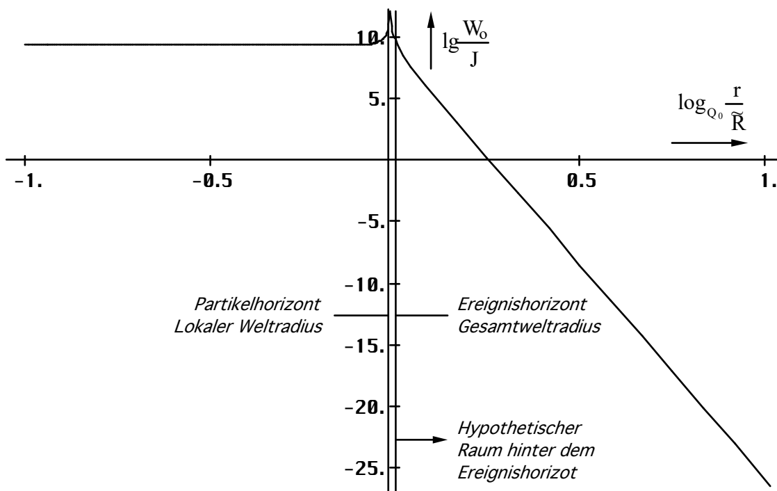
Bild 61 Energie des MINKOWSKISCHEN LINIELEMENTS räumliche Abhängigkeit bis zum Ereignishorizont
