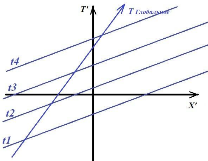
Рис.1 Синее - гиперплоскости АСО для последовательных моментов Глобального Времени Вселенной. Чёрное - оси T' и X' Системы отсчёта Земли.
