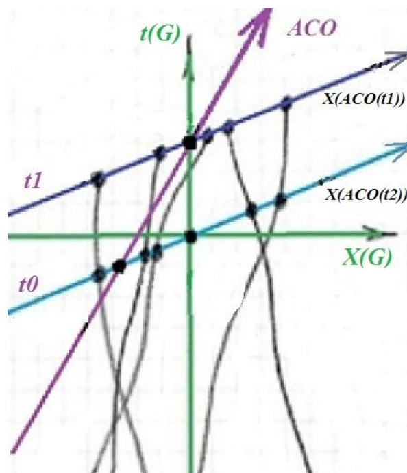
Рис.7. Изображение некоторой части Вселенной в соответствие с гипотезой Абсолютной Системы Отсчёта. Вид из дрейфующей СО Земли.
