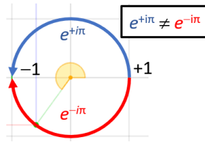
Figure 10: e^{+i\pi} \neq e^{-i\pi}
