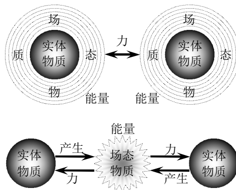
图 12. 实体物质产生场态物质，场态物质对实体物质发生力的作用
