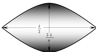
图 10. 光的形状和大小
