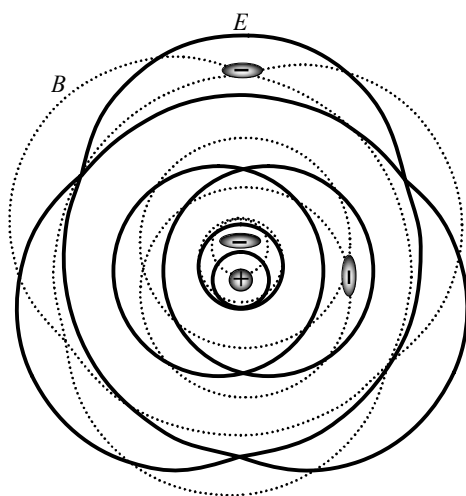
图 5. 类氢原子的广义场波动的形状
