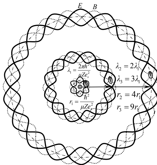
图 3. 类氢原子在三个能级上的电磁场驻波
