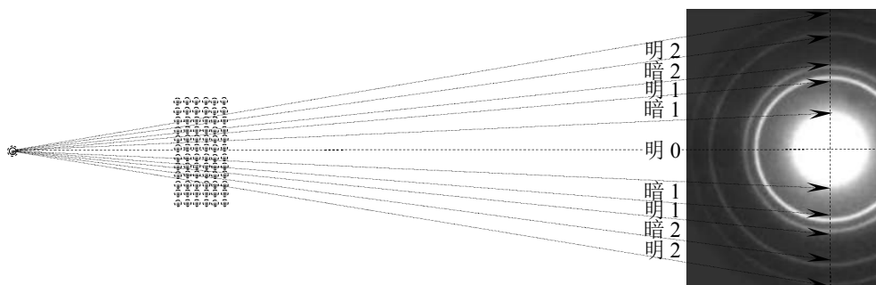
图 16. 戴维孙-革末实验分析图样实例 2
