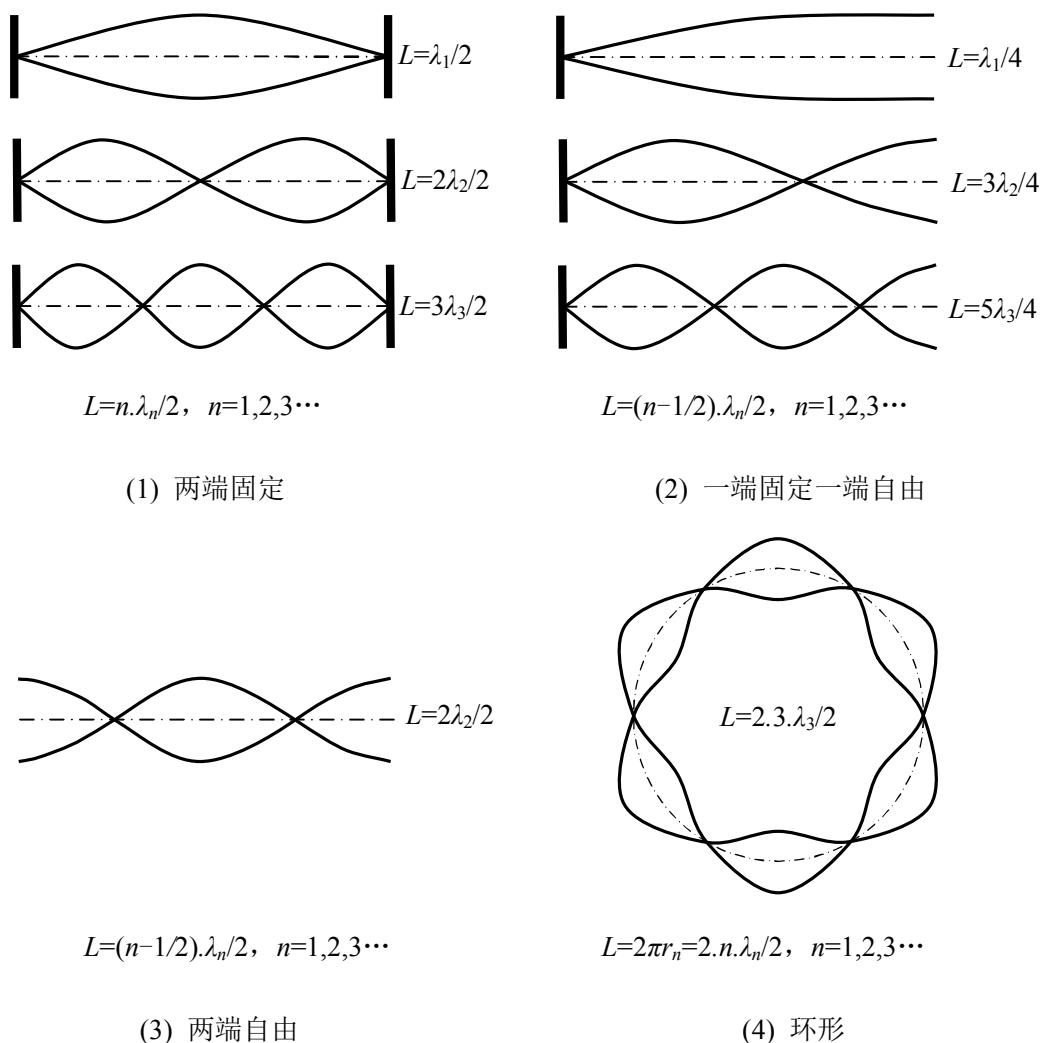
图 7. 几种弦振动驻波模式
