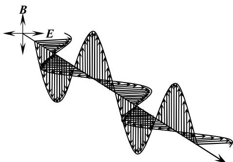
图 9. 电磁波传播图像
