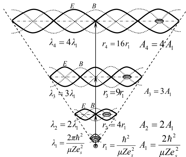
图 4. 类氢原子在四个能级上的电磁场驻波的展开图
