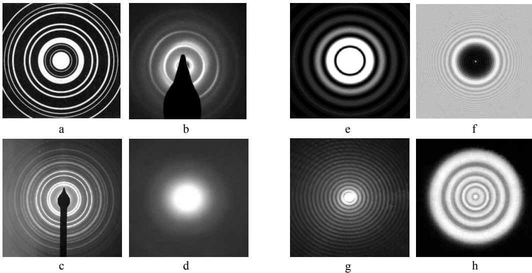
(1)戴维孙-革末实验图样
