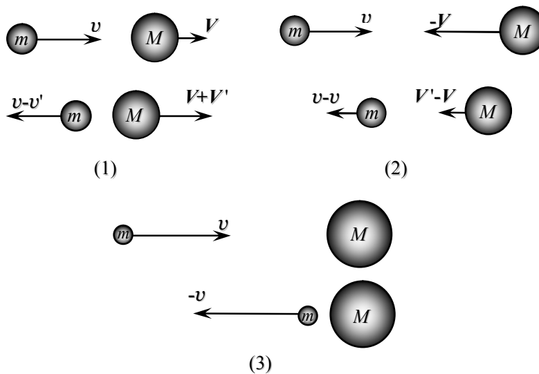
图 2. 动量场在动能势垒中的贯穿
