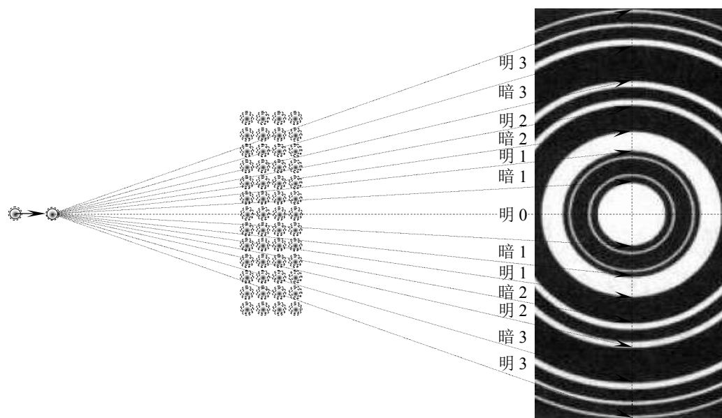
图 15. 戴维孙-革末实验图样分析实例 1
