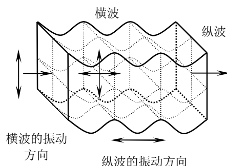
图 8. 体波同时存在横波和纵波
