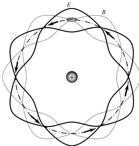
图 6. 电磁场驻波自旋和电子自旋
