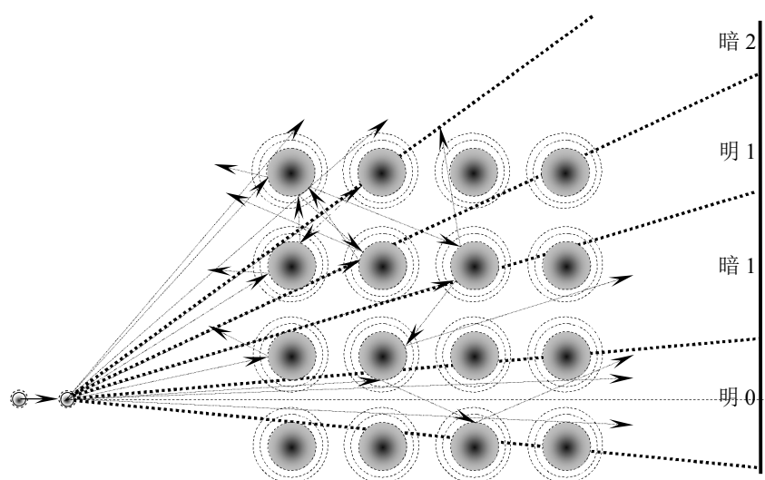
图 14. 戴维孙-革末实验的微观机制
