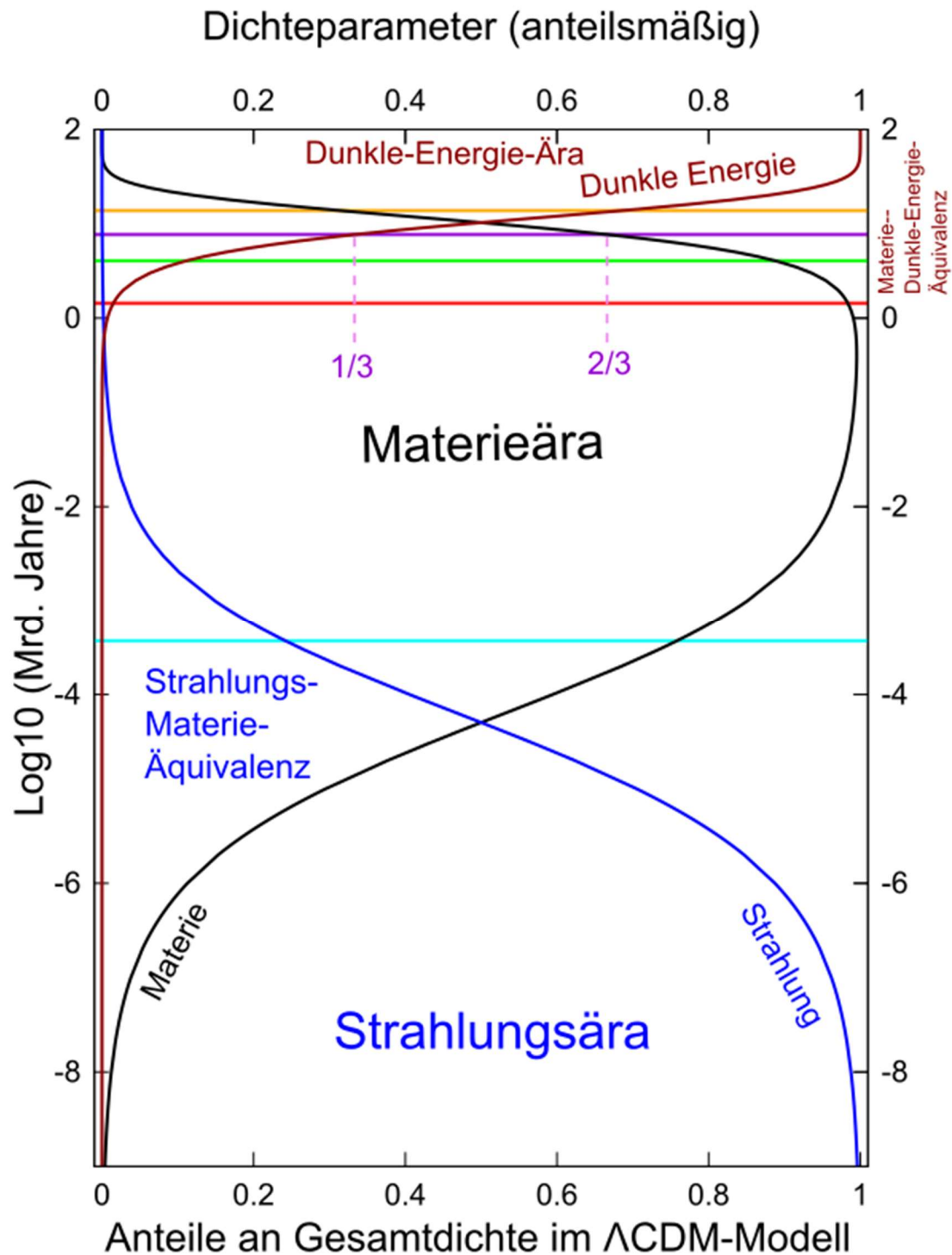
Abbildung 4: Anteilmäßige Dichteparameter in der Geschichte des Universums
