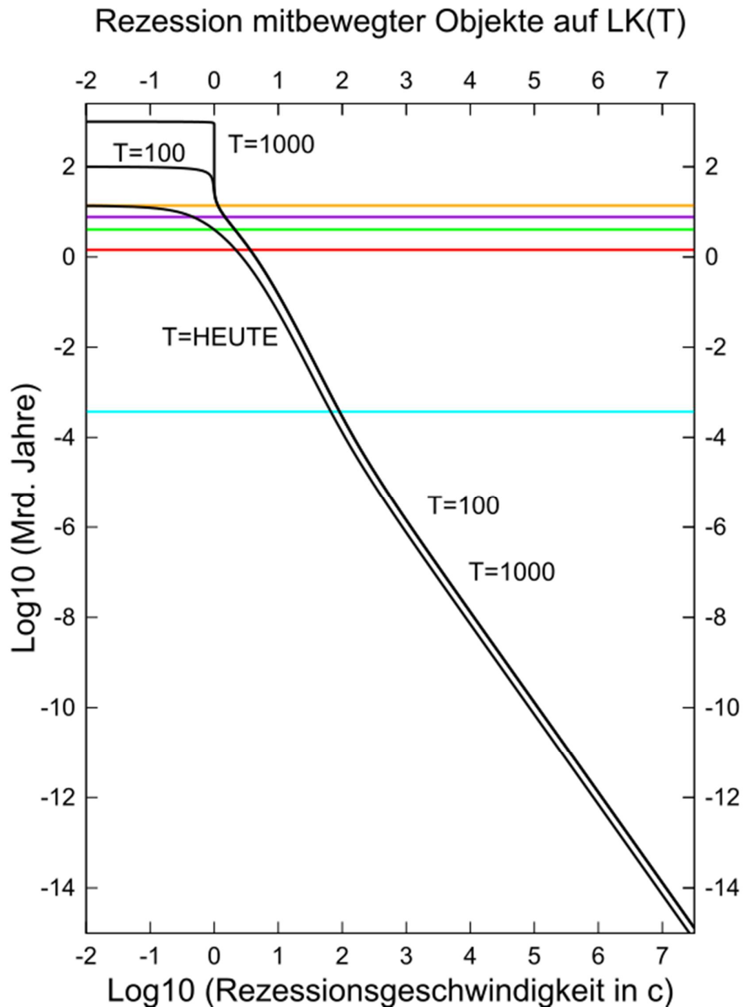
Abbildung 7: Rezession mitbewegter Objekte auf dem jeweiligen Mantel der Lichtkegel LK(HEUTE), LK(100) und LK(1000) in physikalischen Koordinaten
