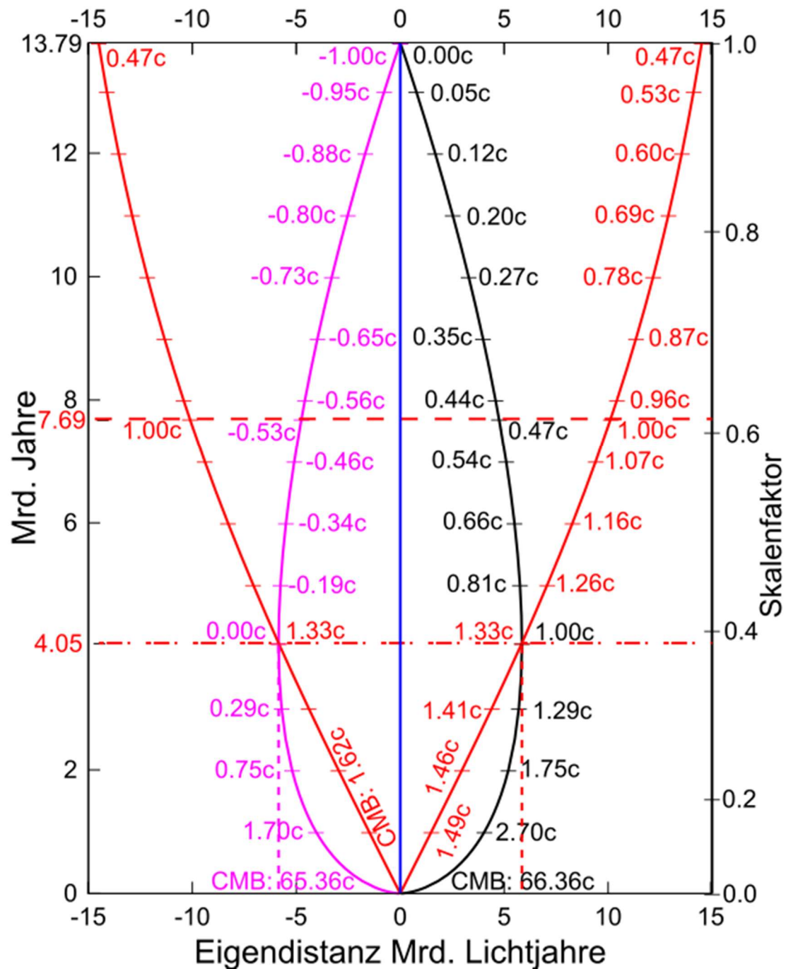
Abbildung 3: Rezessionsgeschwindigkeiten in physikalischen Koordinaten der Oberfläche der Hubblesphäre (rot), von Galaxien auf dem Mantel des Lichtkegels LK(HEUTE) (schwarz) und von auf den Beobachter gerichteten Photonen auf dem Mantel von LK(HEUTE) (magenta). Negative „Rezessionsgeschwindigkeiten“ deuten an, dass sich die entsprechenden Photonen dem Beobachter annähern.
